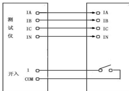
三相反时限接线
