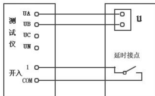
时间继电器接线
