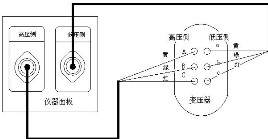
图十八、三相变压器的测试接线
