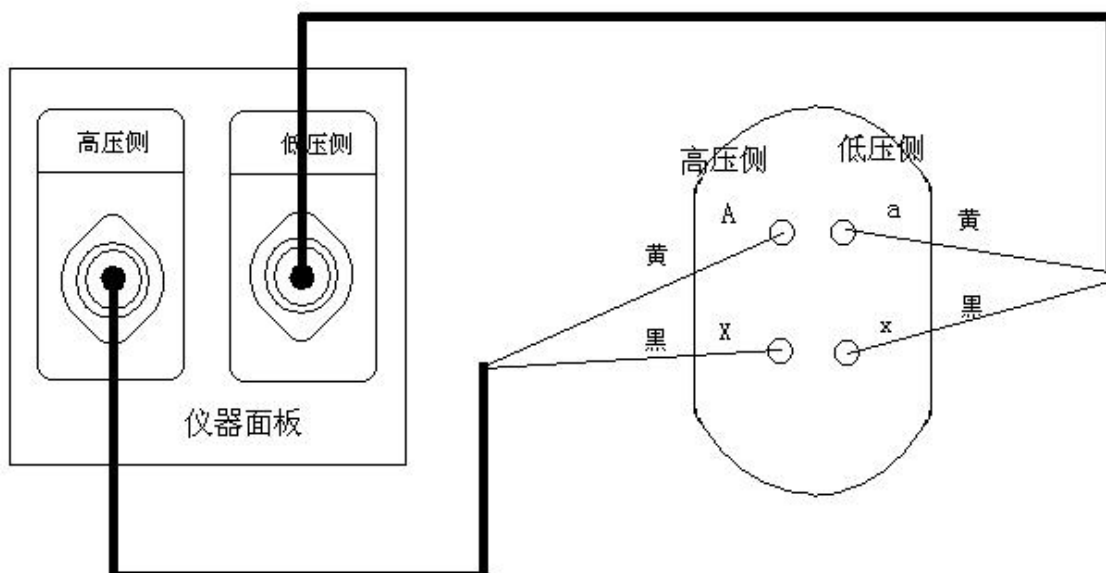
图十九、单相变压器的测试接线
