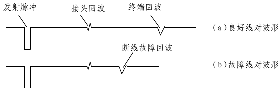
图 11 比较法波形
