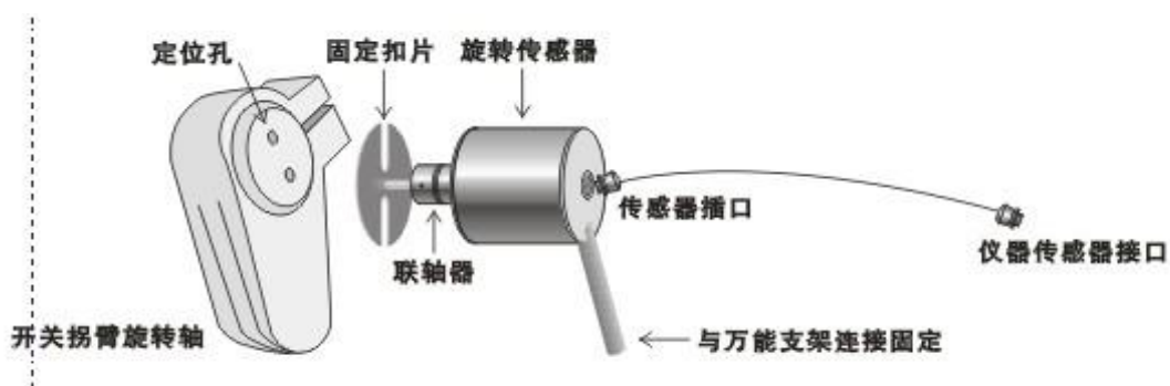
图 13 旋转传感器安装示意图
