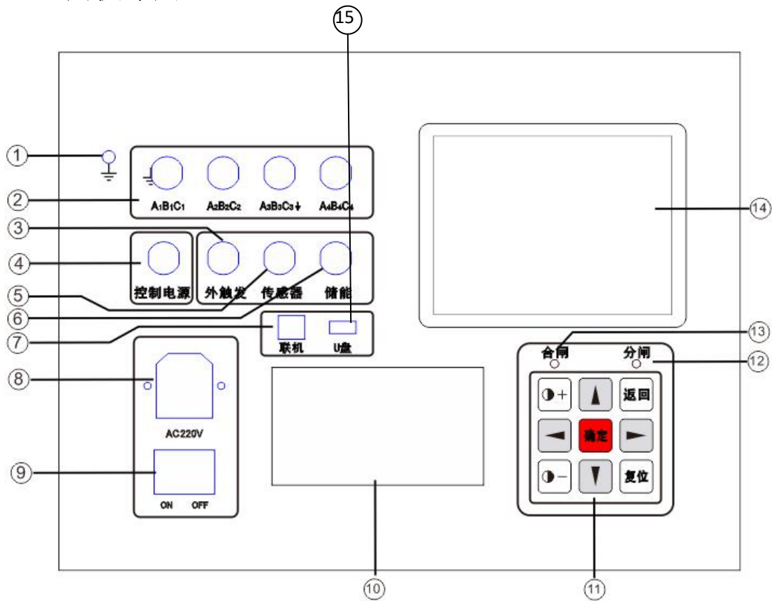
图 1 面板布局图
