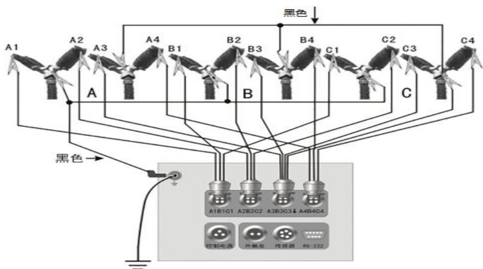
图 11 十二断口接线图
